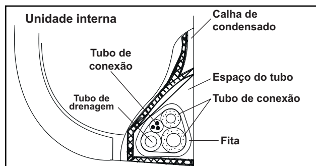
FIGURA 18 - TUBO DE CONEXÕES
