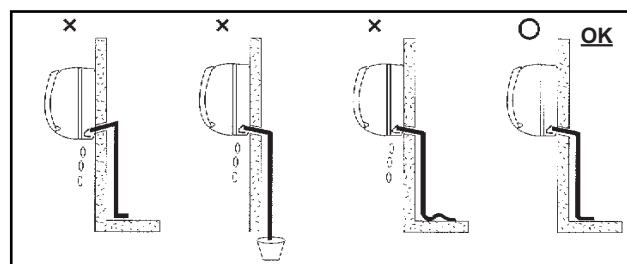
FIGURA 15 - SITUAÇÕES DE DRENAGEM INEFICAZ
