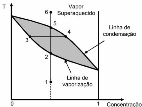
Figura 3.67 - Diagrama Concentração(temperatura)
