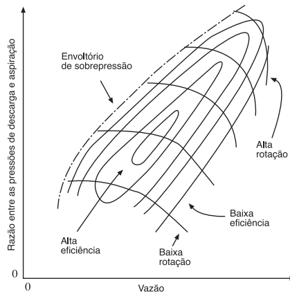
Figura 3.16 - Desempenho de um compressor centrífugo
