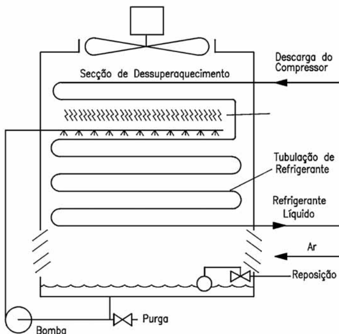
Figura 3.30 - Condensador evaporativo
